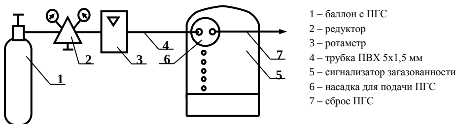
Рисунок Г.1 – Схема для поверки сигнализатора
