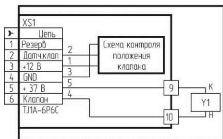
а) XS1 – разъем типа MDN-8FR
