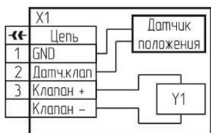
а) с разъемом типа PG1H-1-3
