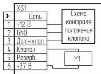
б) с разъемом типа BG5NO3000-UL
