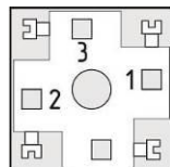
Вилка на кабель PSH2N-1-17, нумерация контактов (вид со стороны пайки)
