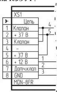
б) XS1 разъем типа TJ1A-6P6C
